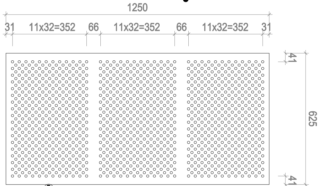
CETRIS ® AKUSTIC B Bohrung Ø 12 mm
