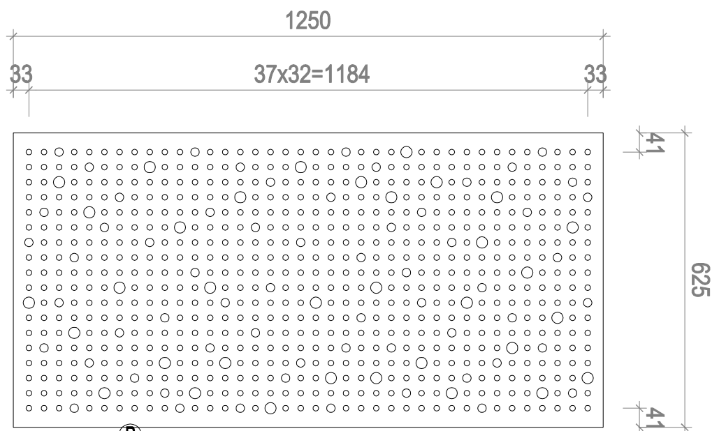
CETRIS ® AKUSTIC D Bohrung %12,18,24 mm
