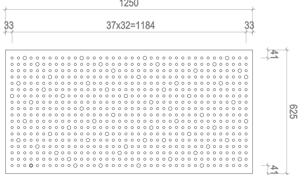
CETRIS ® AKUSTIC C Bohrung Ø 12 a 18 mm
