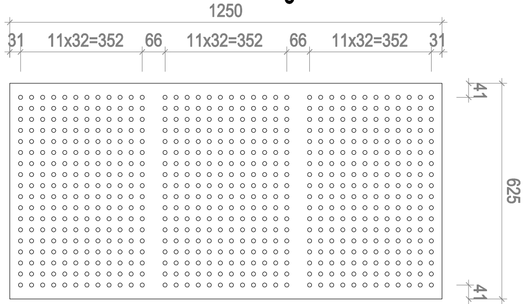
CETRIS ® AKUSTIC A Bohrung Ø 12 mm
